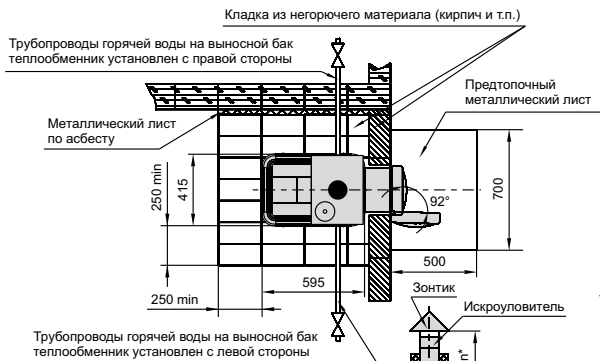
Вид В
